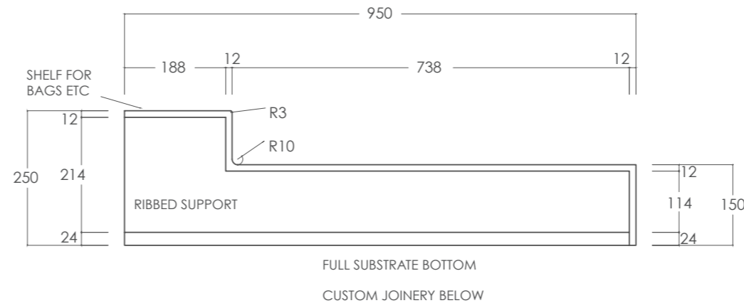
SECTION B SCALE 1:10 A3
