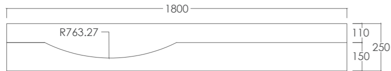
ELEVATION SCALE 1:20 A3
