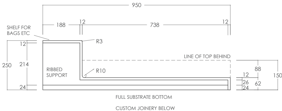
SECTION A SCALE 1:10 A3
