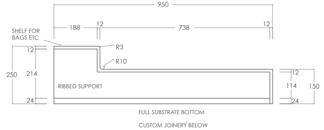
SECTION B SCALE 1:10 A3
