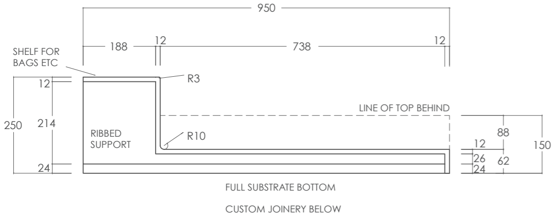
SECTION A SCALE 1:10 A3
