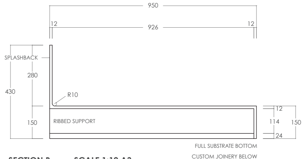
SECTION B SCALE 1:10 A3
