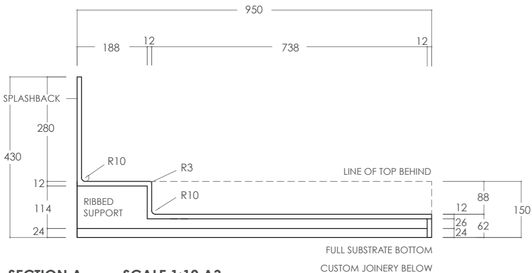
SECTION A SCALE 1:10 A3
