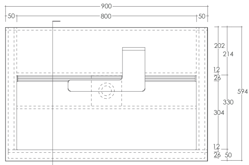
PLAN 1P SCALE 1:10 A3
