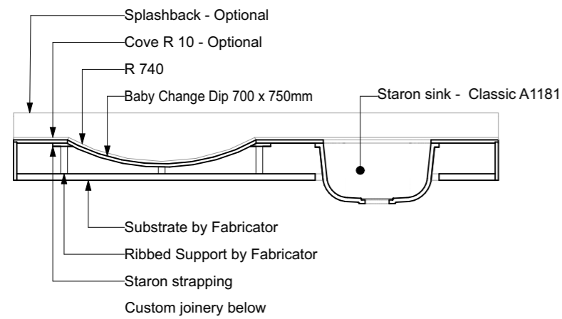
SECTION A-A 1:20
