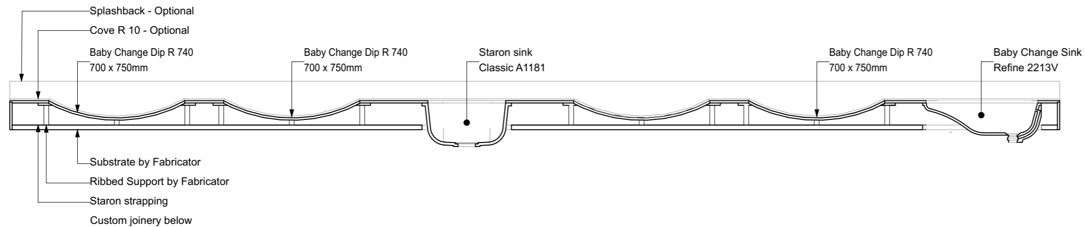
SECTION A-A 1:20
