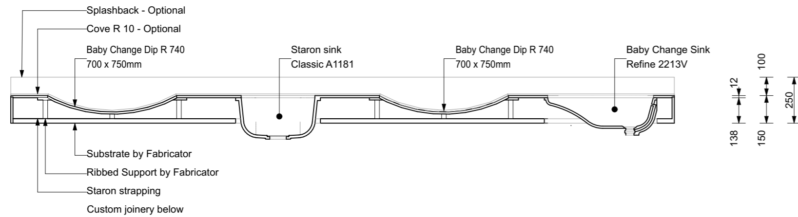
SECTION A-A 1:20
