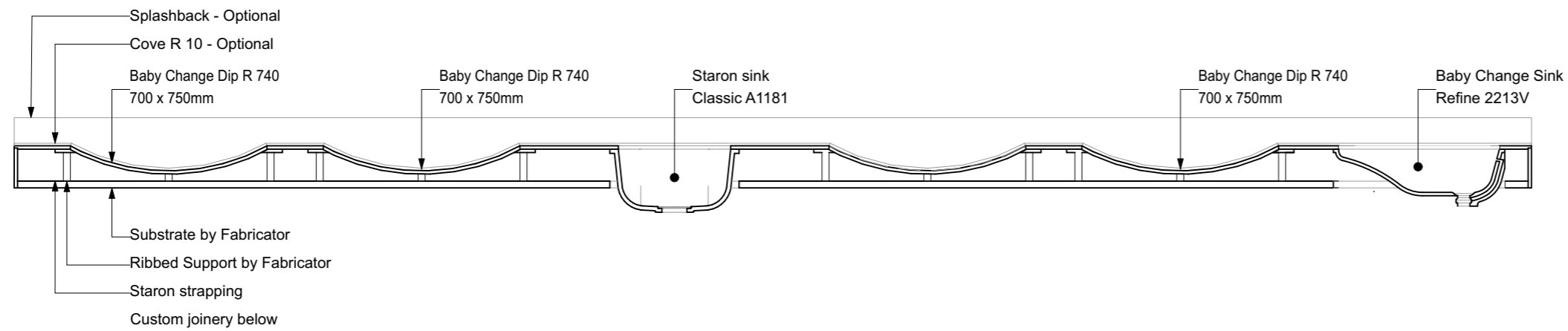
SECTION A-A 1:20
