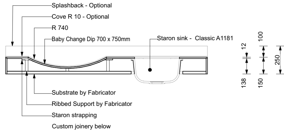
SECTION A-A 1:20
