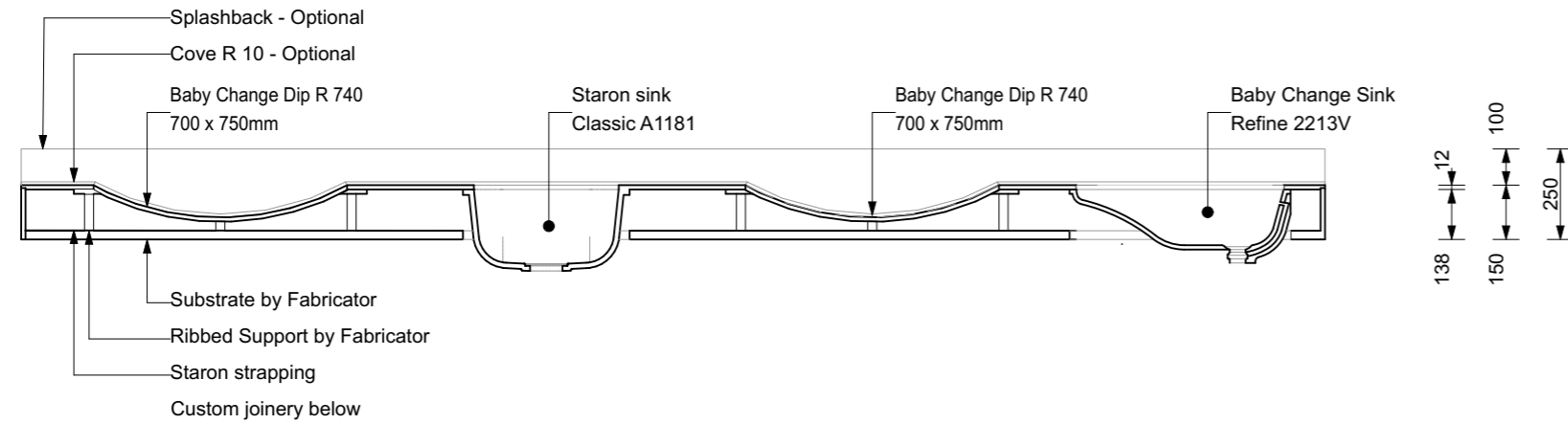
SECTION A-A 1:20
