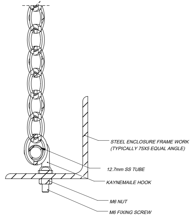
SECTION B-B SCALE 1 : 2
